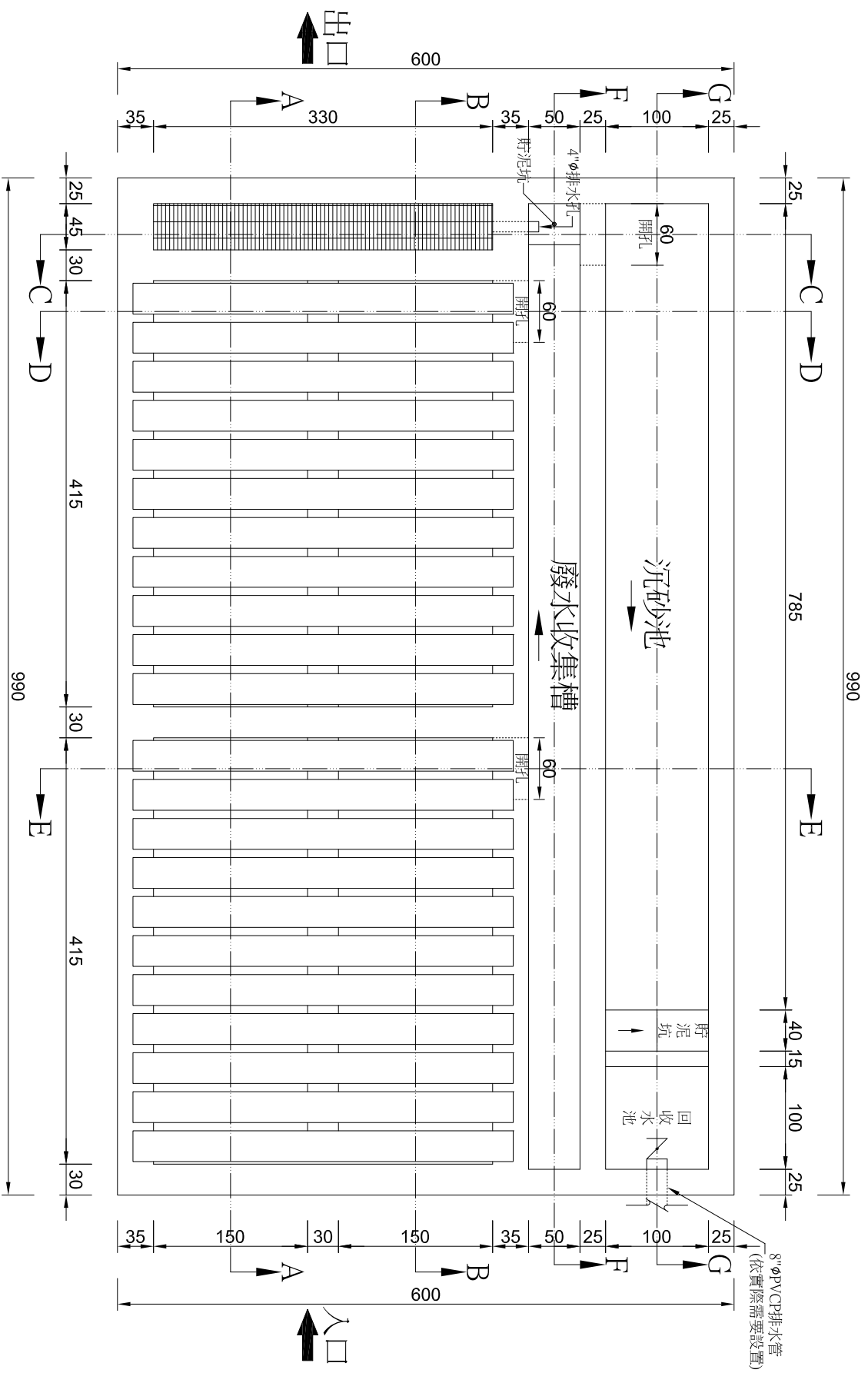
標準型洗車台平面圖
